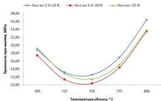
Рис. 1. Зависимость прочности при сжатии от температуры обжига
