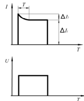
Рис. 3. Эпюры
