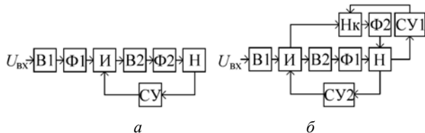
Рис. 1. Структурная электрическая схема традиционного преобразователя – а; структурная схема преобразователя с введенным накопительным компонентом – б
