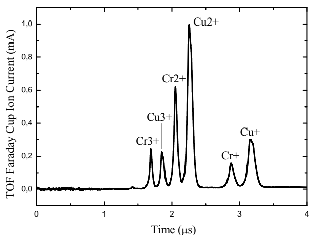
Рис. 3. Спектр состава плазмы вакуумной дуги для электродов из CuCr-50/50. Плотность тока – 2,5 кА/см 2 . Момент измерения – через 150 мкс после инициирования вакуумной дуги
