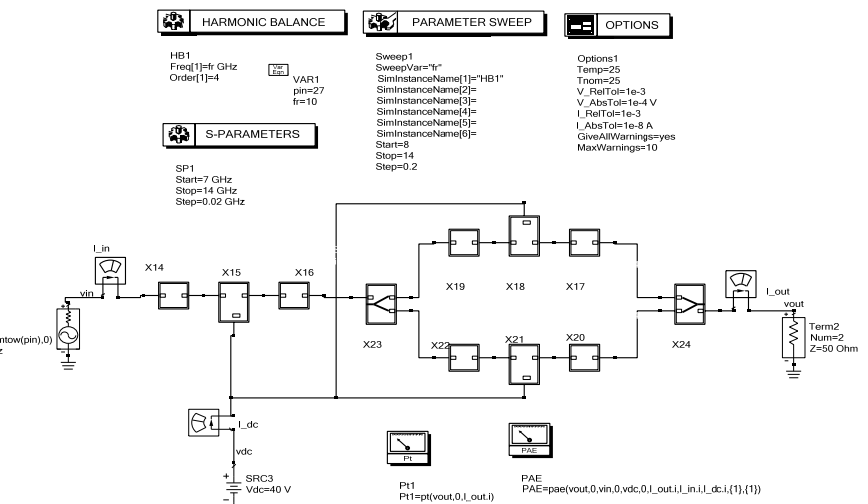
Рис. 9. Общая схема для моделирования в САПР
