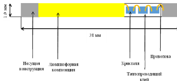
Рис. 2. Конструкция светодиодного излучающего элемента
