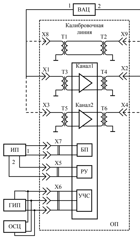
Рис. 1. Схема измерительной установки
