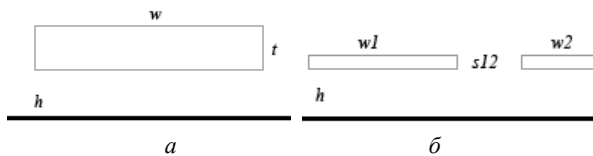
Рис. 1. Примеры одиночной (а) и связанных (б) линий передачи
