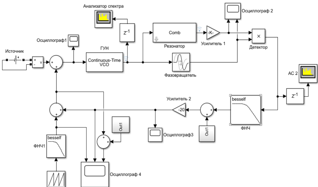
Рис. 3. Структурная схема интерференционной САР ОЭАГ
