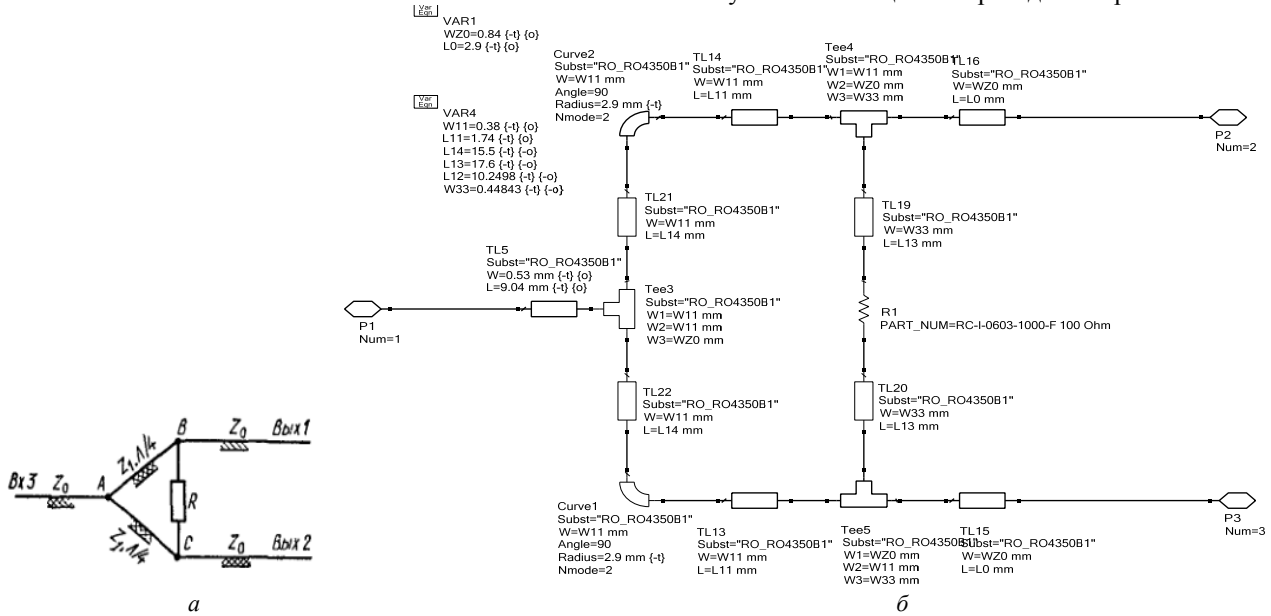
Рис. 6. Электрическая схема (а) моста Уилкинсона и схема в САПР ADS (б)
