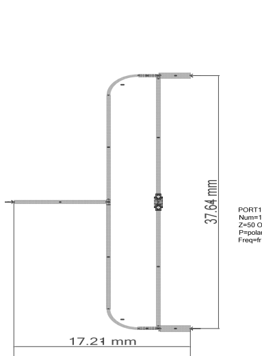
Рис. 8. Топология моста Уилкинсона
