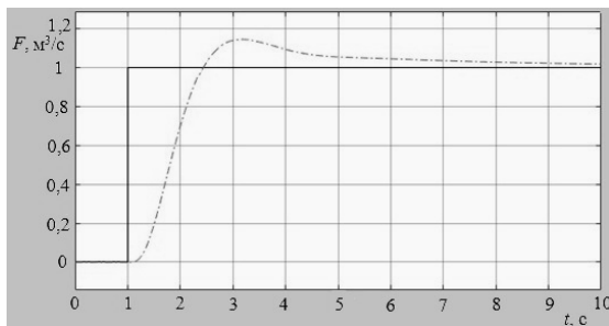
Рис. 4. Результат моделирования с использованием ПИД-регулирования
