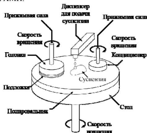
Рис. 1. Схема установки ХМП
