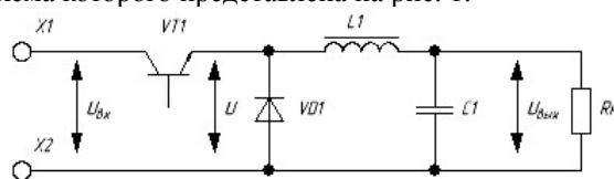
Рис. 1. Преобразователь понижающего типа
