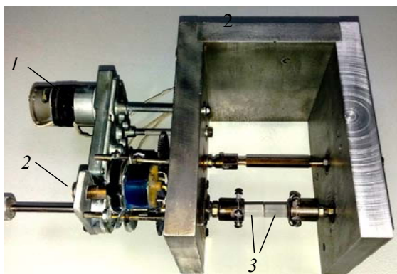
Рис. 2. Модернизированная система вращения: 1 – электромотор для вращения образцов; 2 – система сближения образцов; 3 – свариваемые образцы
