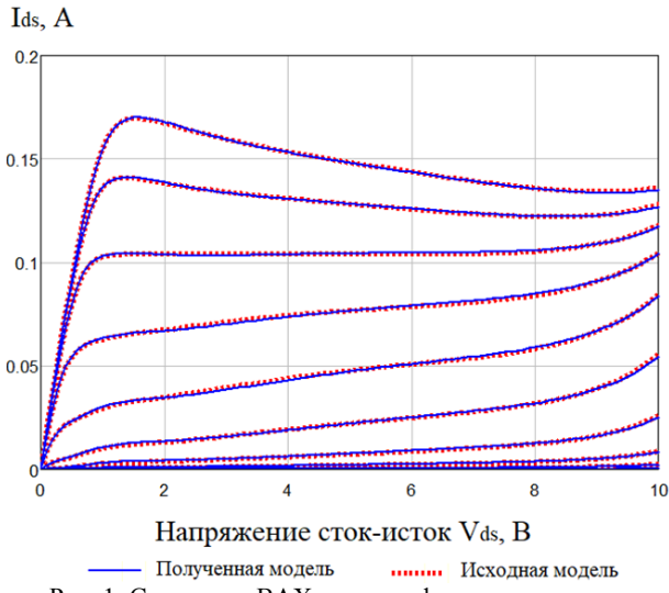
Рис. 1. Сравнение ВАХ при верификации методики
