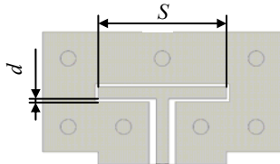
Рис. 3. Пример топологии тестового двухполюсника
