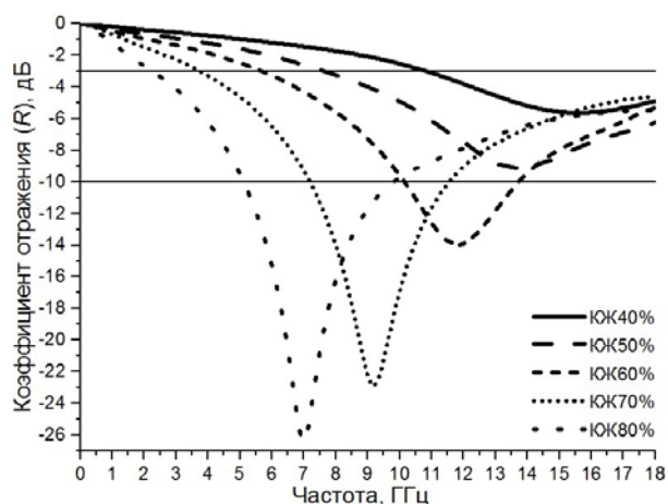
Рис. 2. Частотная зависимость коэффициента отражения для различных концентраций карбонильного железа
