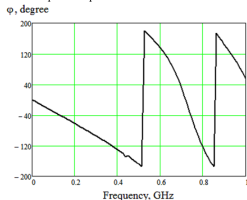
Рис. 13. Частотная зависимость вносимого фазового сдвига корректором ГВЗ
