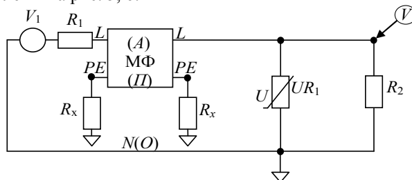
Рис. 5. Схема дифференциального включения МФ и варистора
