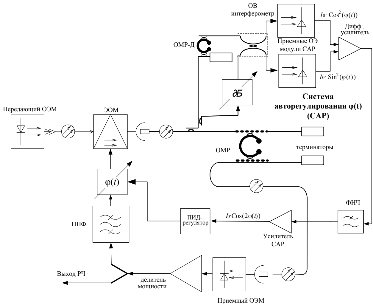
Рис. 2. Схема ОЭАГ с комбинированной стабилизацией частоты на основе оптического интерферометра
