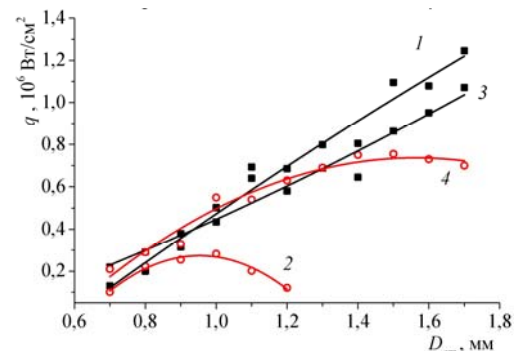
Рис. 2. Зависимости плотности мощности q электронного пучка от диаметра эмиссионного канала D_{em} для различных давлений P и рода газа: воздух – 1, 2 и P = 4 и 8 Па соответственно; гелий – 3, 4 и P = 10 и 30 Па соответственно
