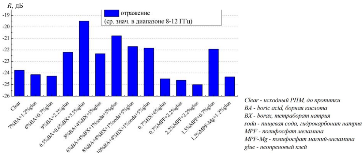
Рис. 2. Результаты измерения уровня отражения
