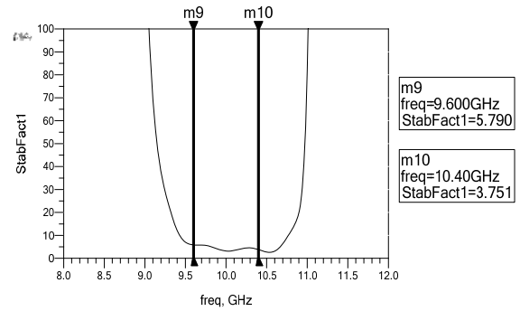
Рис. 12. Стабильность усилителя
