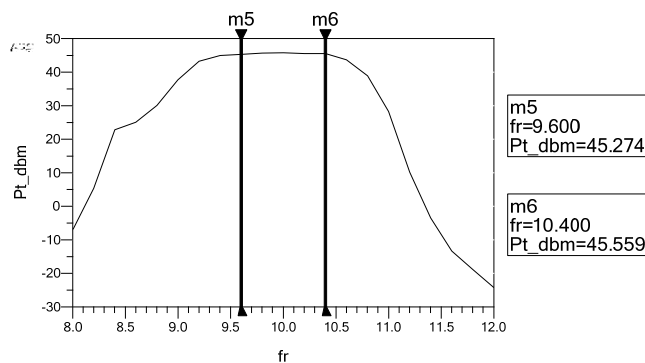
Рис. 11. График мощности
