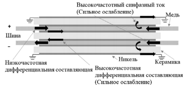
Рис. 5. Фильтр ЭМП на основе линии передачи
