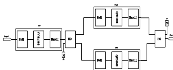
Рис. 9. Структурная схема СВЧ-усилителя мощности
