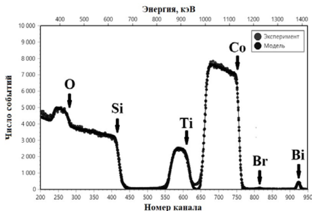
Рис. 6. Спектр POP пленки, содержащей титан, кобальт, бром и висмут
