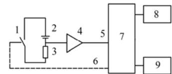
Рис. 2. Функциональная схема прибора
