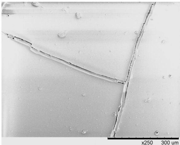
Рис. 3. Фотография поверхности полипропиленового образца с полученным покрытием. Количество импульсов N = 100 . Параметры эксперимента: I_e = 20 А; U_a = 9 кВ; \tau_d = 5 мс; B_1 = 0,6 мТ; B_2 = 4,2 мТ
