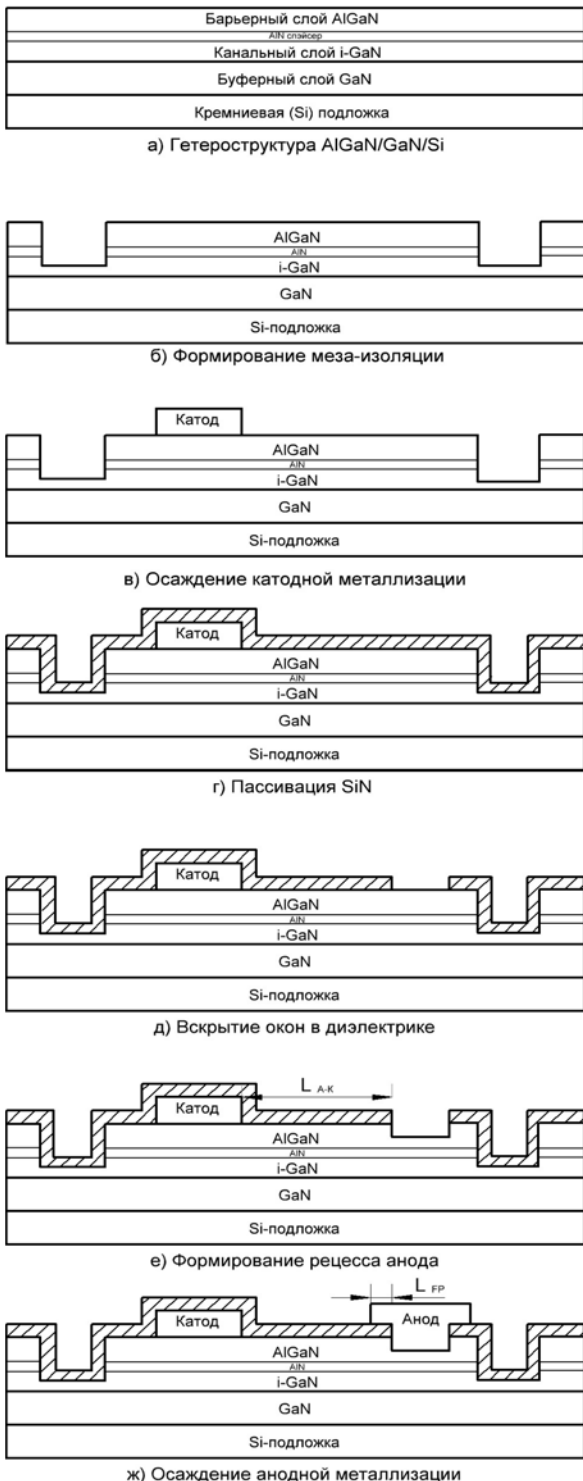
Рис. 1. Техмаршрут изготовления AlGaIn/GaN-диодов
