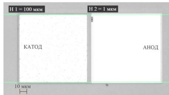
Рис. 2. Микроскопическое изображение GaN ДБШ
