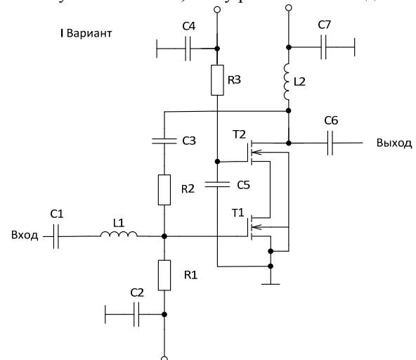
Рис. 1. Принципиальная схема БУ
