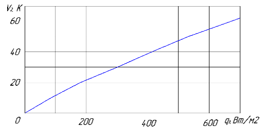
Рис. 2. Зависимость перегрева нагретой зоны от удельной мощности рассеивания
