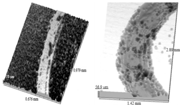
Рис. 3. Фотография трека при измерении триботехнических характеристик
