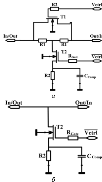
Рис. 1. Ячейка Т-типа – а; ячейка с одним транзистором – б
