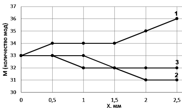
Рис. 3. Модовый состав волноводных каналов с учетом амплитудной (1), фазовой (2) и амплитудно-фазовой (3) неоднородности записывающего поля
