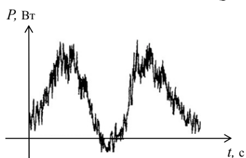
Рис. 1. Ваттметрограмма
