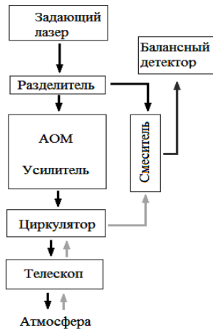
Рис. 1. Схема ИКДЛ
