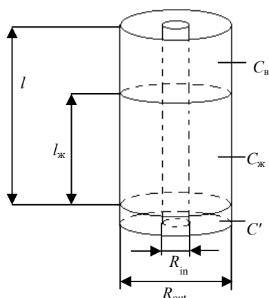
Рис. 1. Составляющие емкости измерительной ячейки
