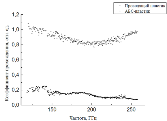
Рис. 2. Частотная зависимость коэффициента прохождения АБС и токопроводящего пластика
