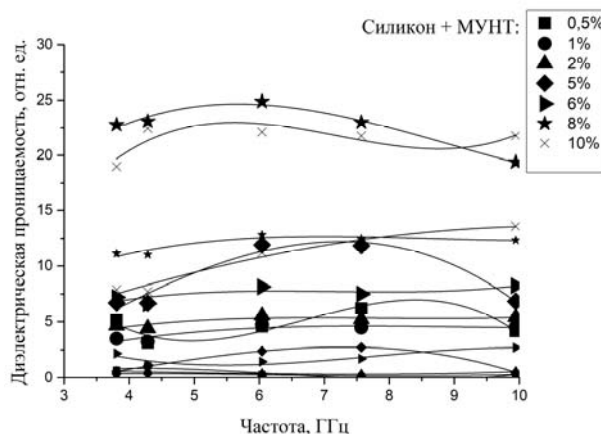
Рис. 1. Частотные зависимости диэлектрической проницаемости композитов на основе силикона и МУНТ
