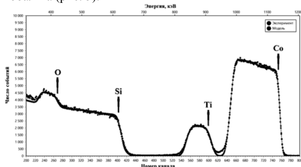
Рис. 5. Спектр POP пленки, содержащей титан и кобальт
