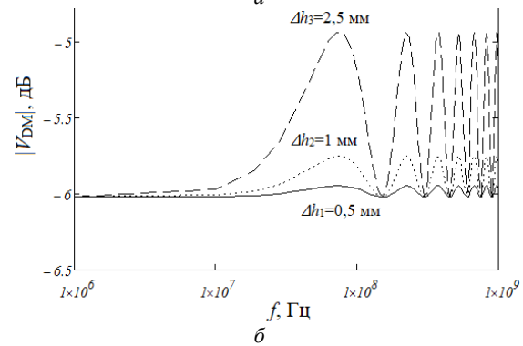
Рис. 2. Частотные зависимости ДМ на конце ДЛ из [1] (а) и по разработанному алгоритму (б) для \Delta h = 2,5 (пунктирные кривые); \Delta h = 1 (пунктирно-точечные кривые); \Delta h = 0,5 (сплошные кривые) мм
