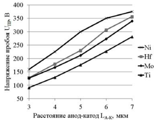
Рис. 6. Обратная ветвь ВАХ изготовленных диодов
