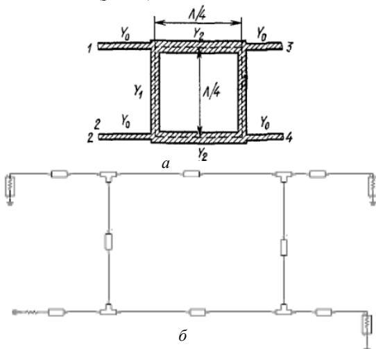
Рис. 1. Топология (а) НО и схема в САПР ADS (б)
