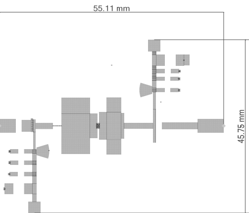
Рис. 5. Топология выходного усилителя мощности
