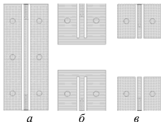
Рис. 2. Топология калибровочных мер: a – линия передачи; b – холостой ход; v – короткое замыкание
