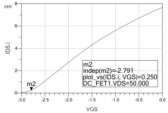
Рис. 5. Передаточная ВАХ транзистора QPD1008
