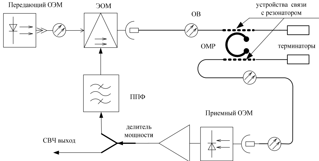
Рис. 1. Структурная схема ОЭАГ на основе ОМП
