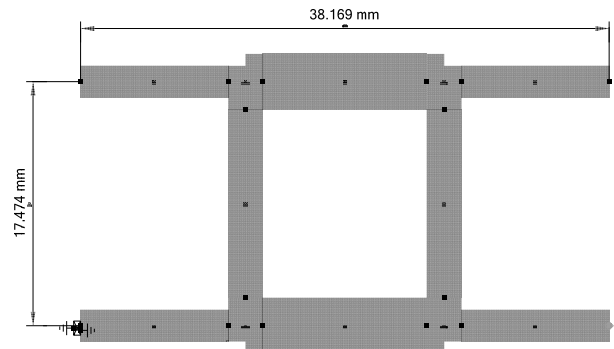
Рис. 3. Топология НО
